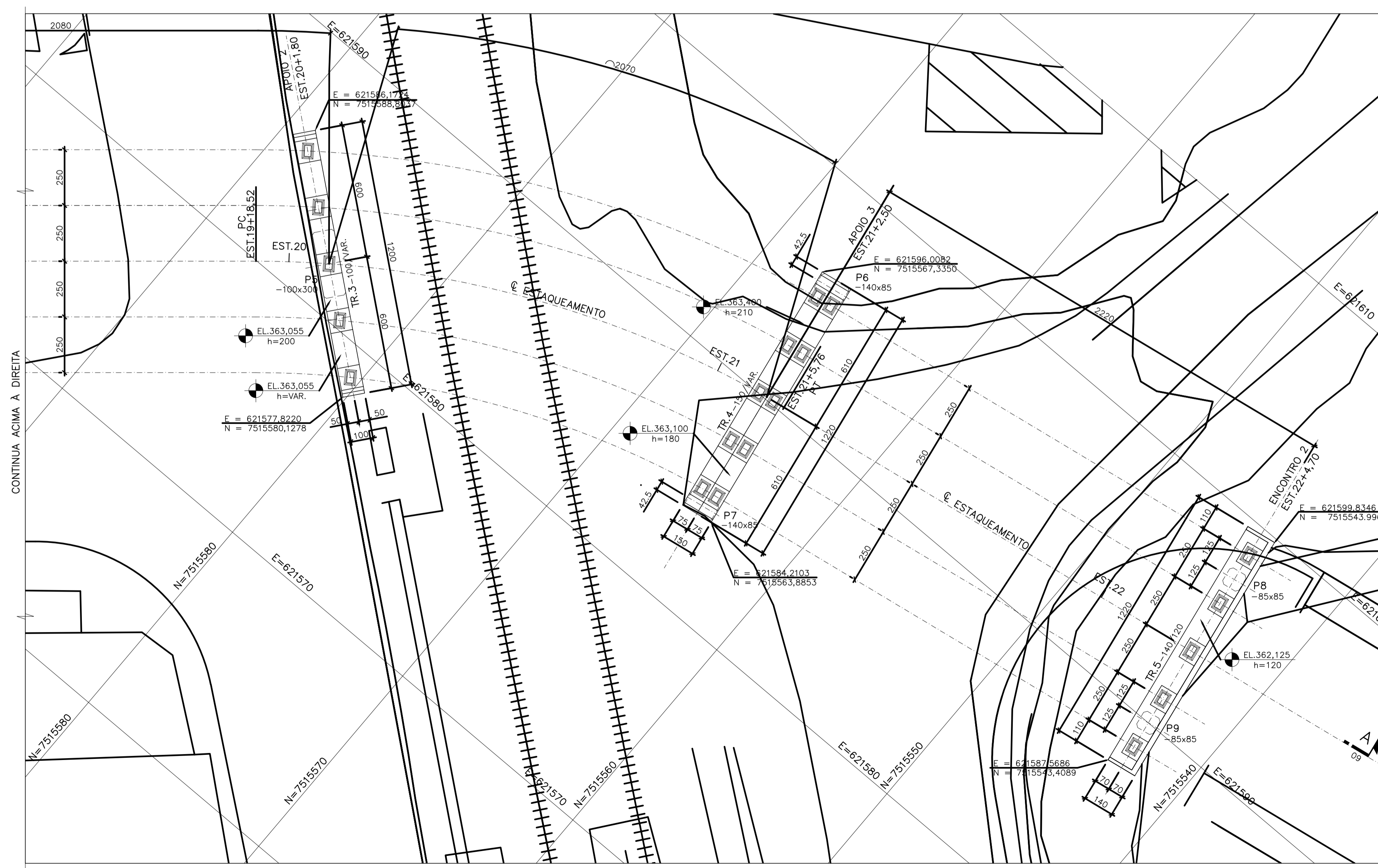
MESOESTRUTURA - PLANTA (2ª PARTE) ESC 1:125
