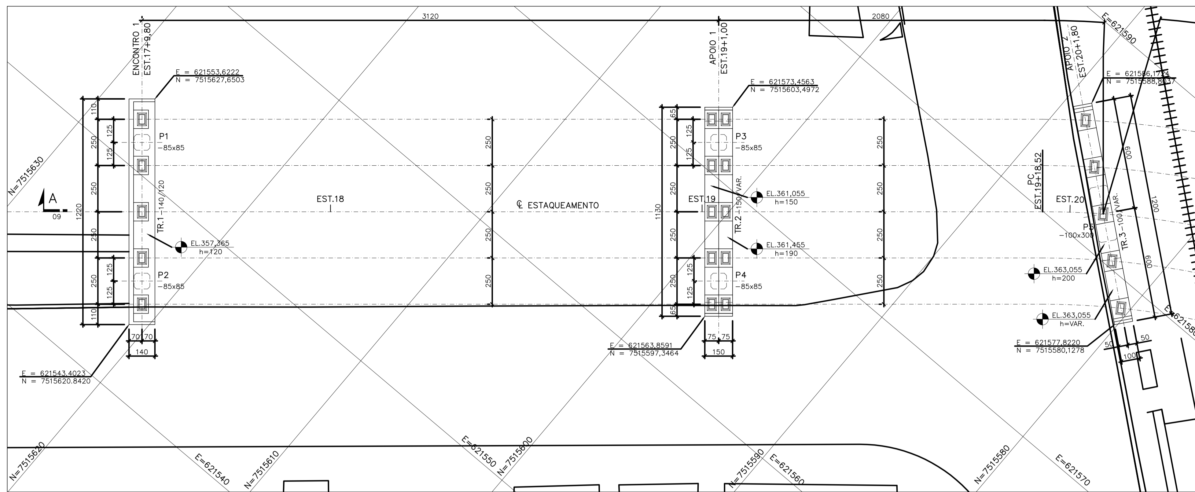
MESOESTRUTURA - PLANTA (1ª PARTE) ESC 1:125
